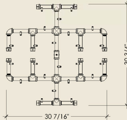
TOP ELEVATION
