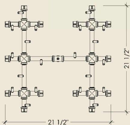
TOP ELEVATION
