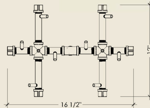
TOP ELEVATION
