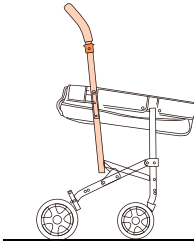
양쪽의 폴딩 레버를 동시에 당기면서 핸들을 앞으로 들어올리듯 밀어주세요
