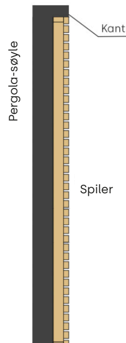
Sidevisning
