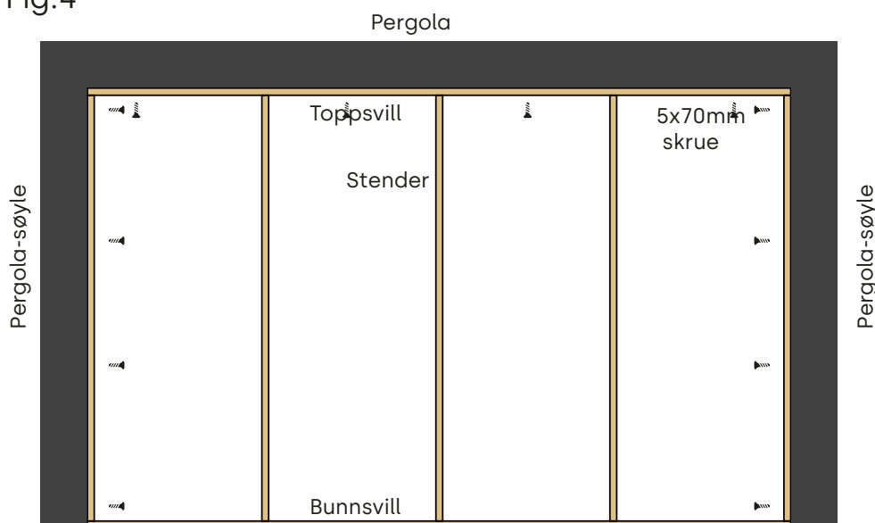
Frontvisning
