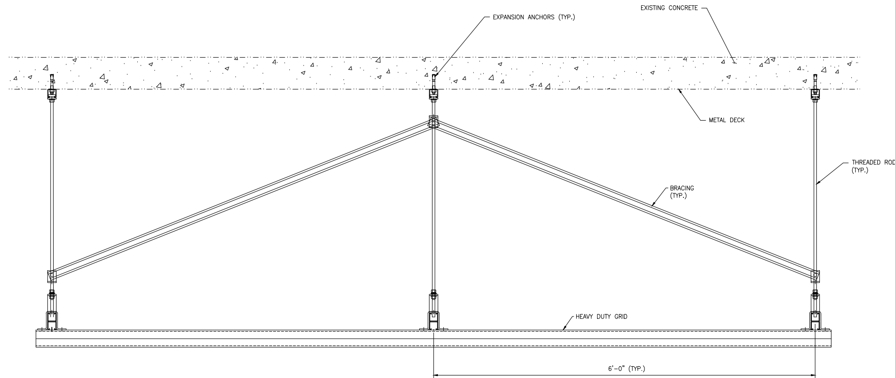
VIEW 1 SCALE: 1 1/2"=1'-0"
