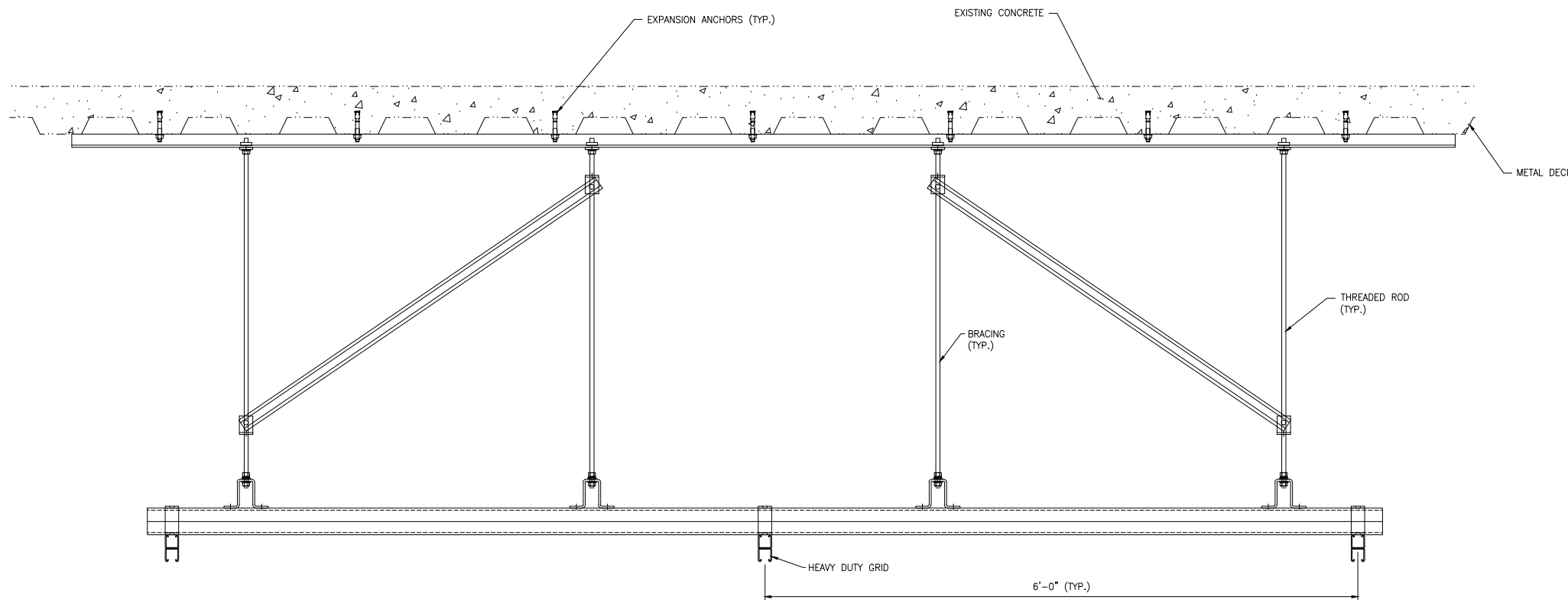
VIEW 2 SCALE: 1 1/2"=1'-0"
