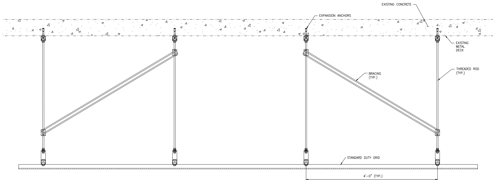
VIEW 1 SCALE: 1 1/2"=1'-0"
