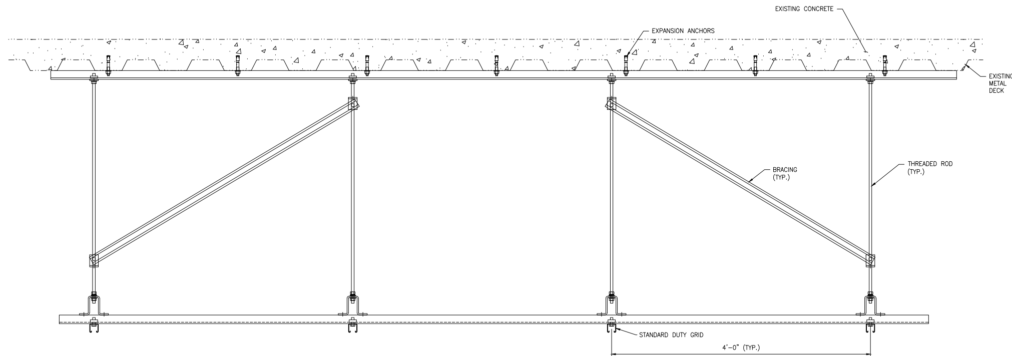
VIEW 2 SCALE: 1 1/2"=1'-0"
