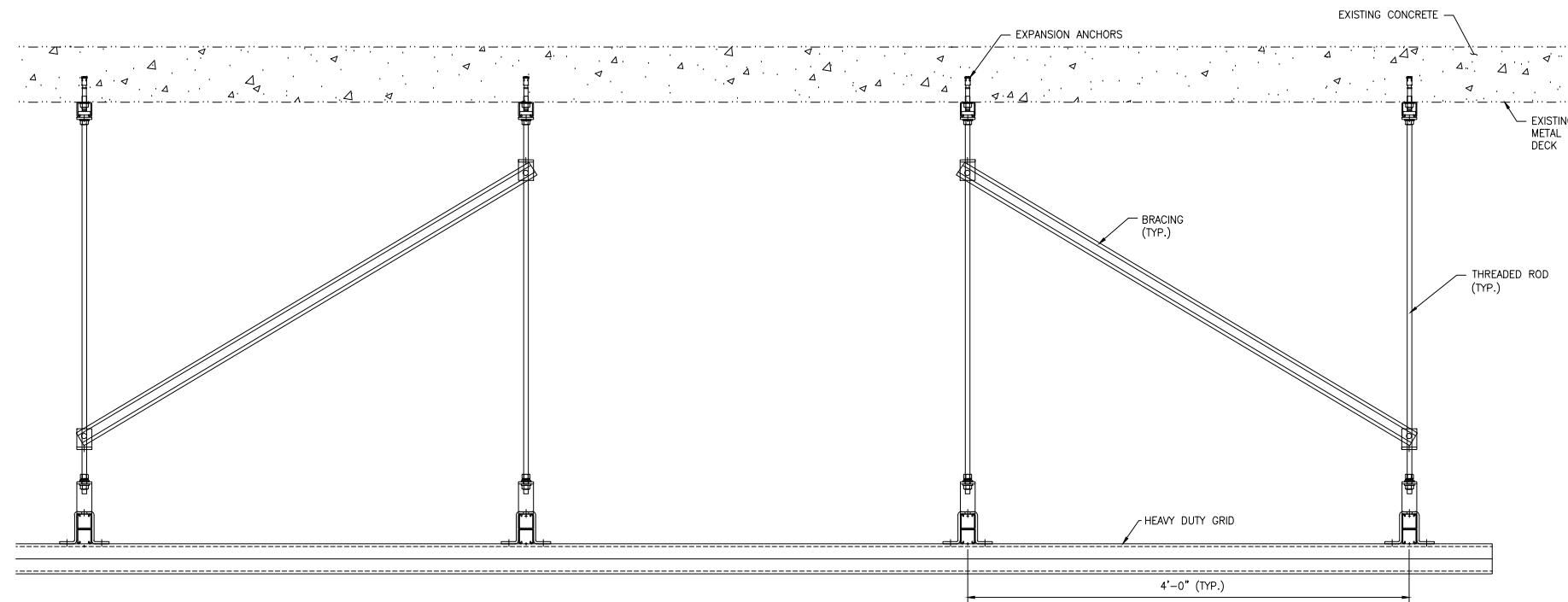
VIEW 1 SCALE: 1 1/2"=1'-0"
