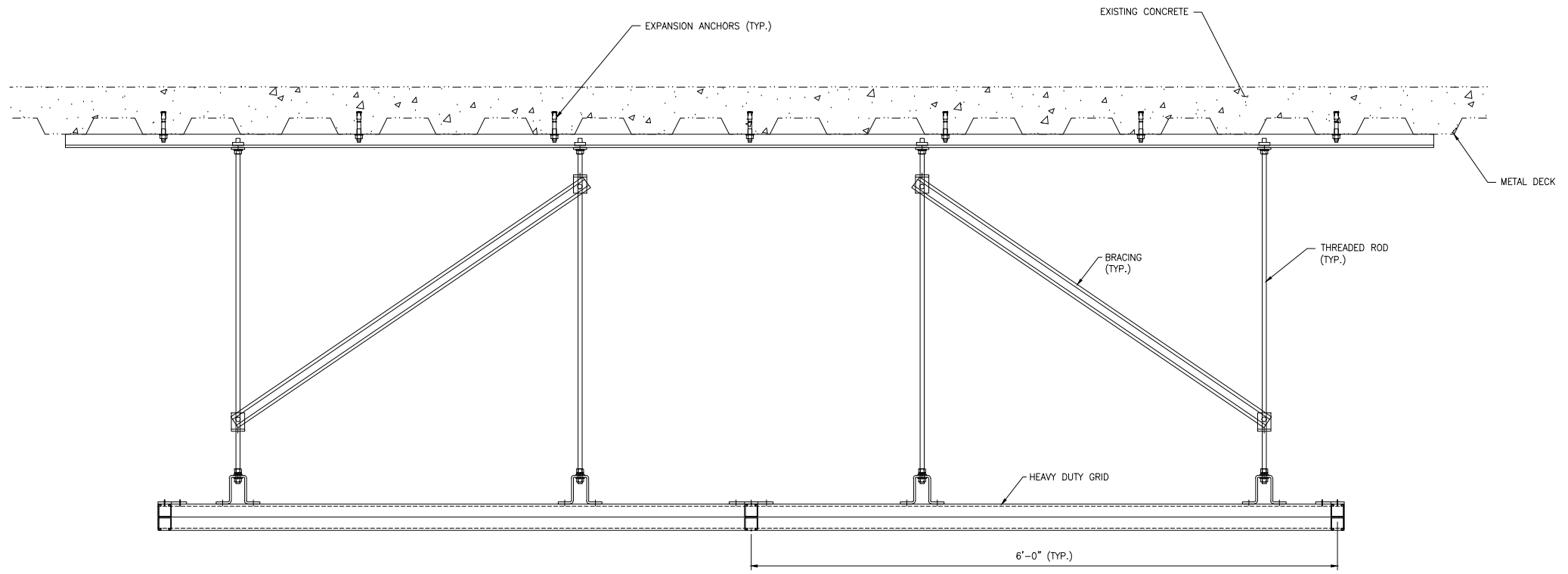
VIEW 2 SCALE: 1 1/2"=1'-0"
