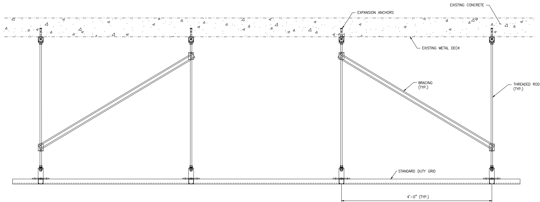
VIEW 1 SCALE: 1 1/2"=1'-0"
