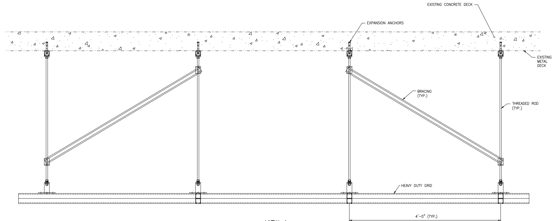
VIEW 1 SCALE: 1 1/2"=1'-0"
