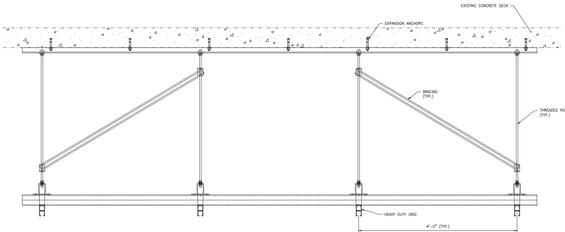
VIEW 2 SCALE: 1 1/2"=1'-0"
