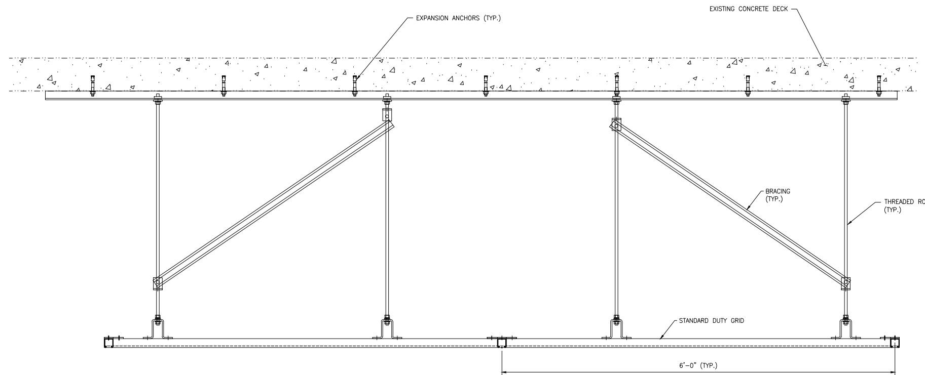
VIEW 2 SCALE: 1 1/2"=1'-0"
