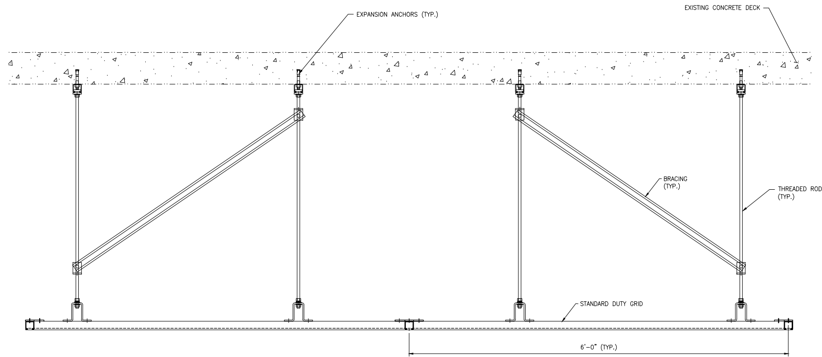
VIEW 1 SCALE: 1 1/2"=1'-0"
