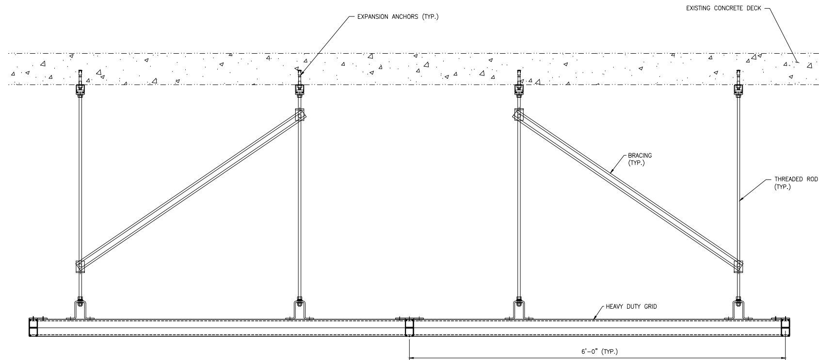
VIEW 1 SCALE: 1 1/2"=1'-0"
