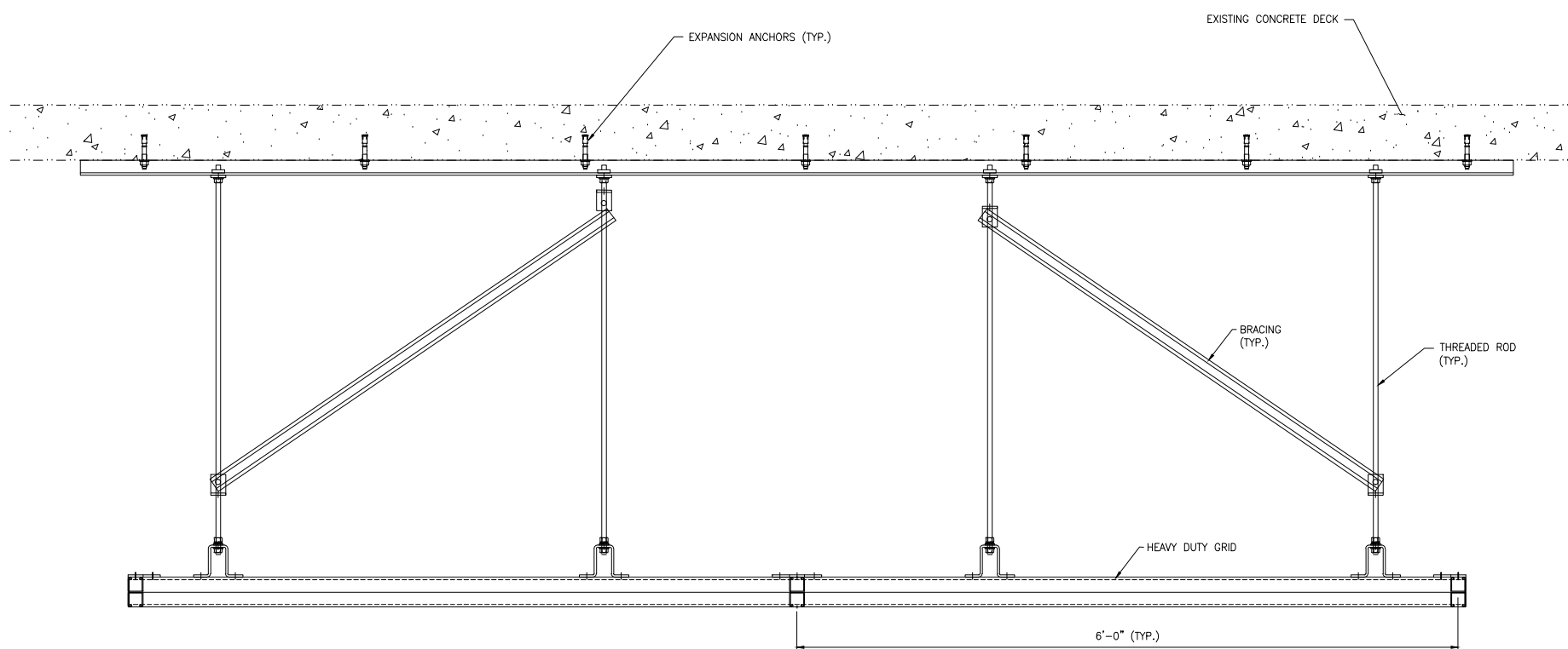
VIEW 2 SCALE: 1 1/2"=1'-0"
