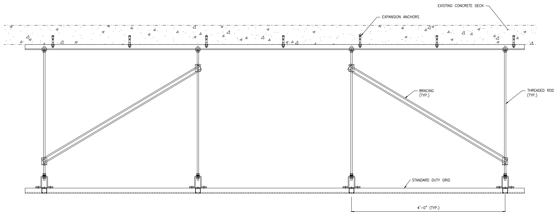
VIEW 2 SCALE: 1 1/2"=1'-0"
