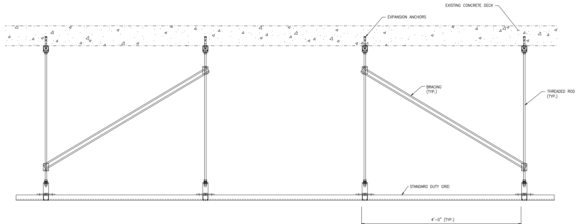
VIEW 1 SCALE: 1 1/2"=1'-0"
