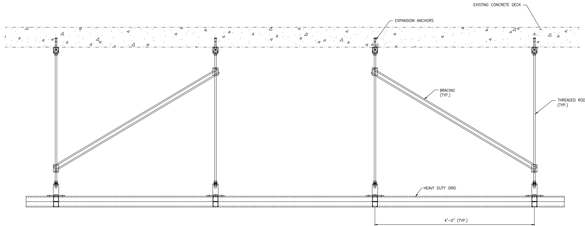
VIEW 1 SCALE: 1 1/2"=1'-0"
