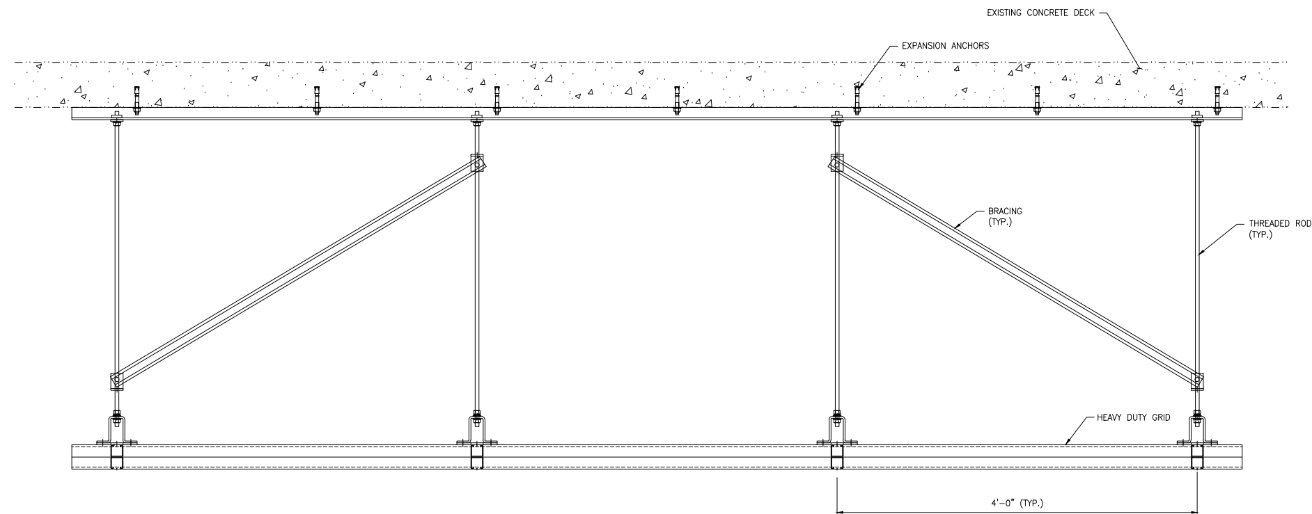
VIEW 2 SCALE: 1 1/2"=1'-0"
