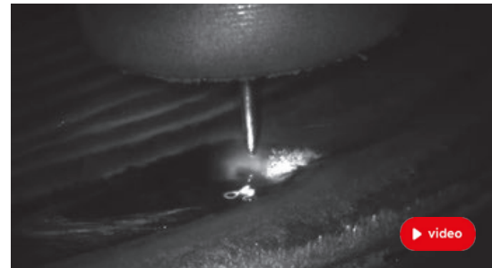
WAAM (RAMLAB)
