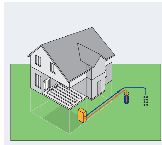
Wärmequelle Grundwasser
