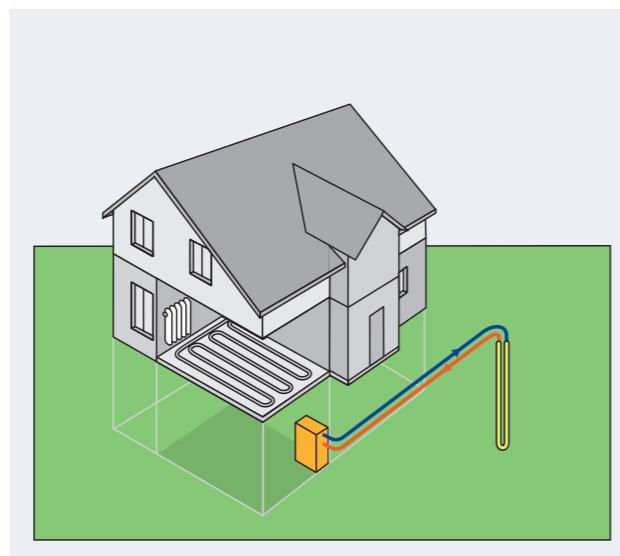
Wärmequelle Erdreich
