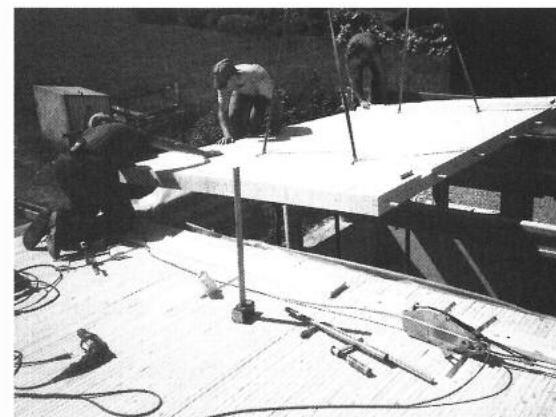
Holzverbunddecke
