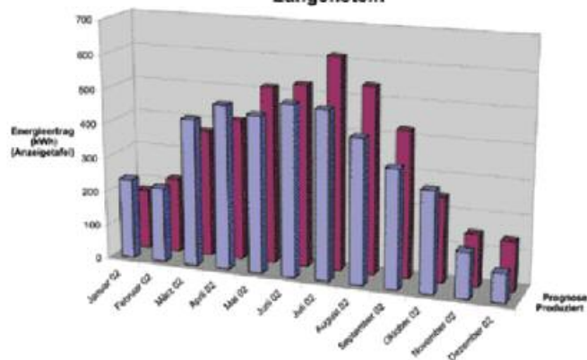
Prognose und Ertrag der 4.8 kWp Fotovoltaikanlage Längenstein
