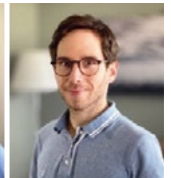
Roger Emmenegger
