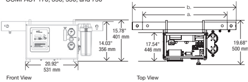
Front View Top View a. PRO Mini 350 & 550: 37.94" / 964 mm | b. PRO Mini 750: 46.94" / 1192 mm
