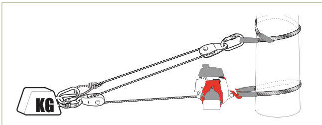
MECHANISCH VOORDEEL X 3
