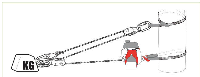
MEKANISK FÖRDEL X 3
