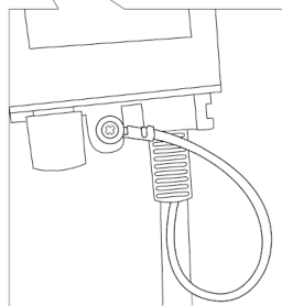
Erdungskabel anschrauben
