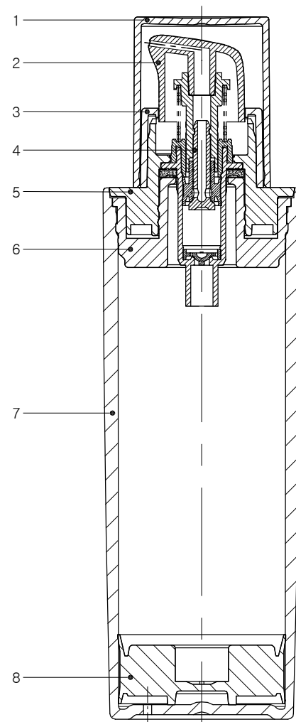
SECTION A-A'
