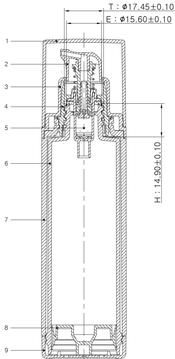
SECTION A-A'
