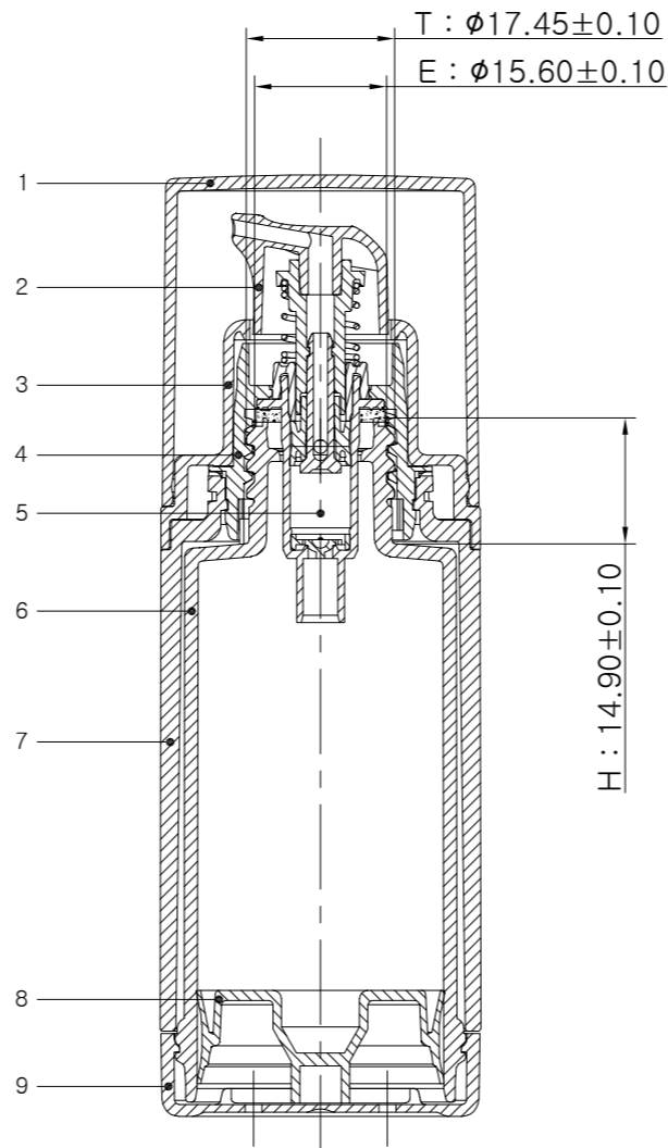
SECTION A-A'
