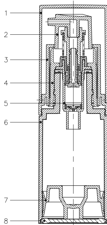
SECTION A-A'
