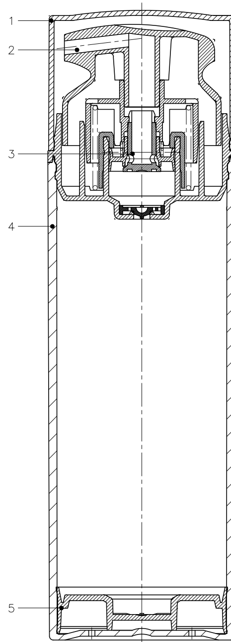
SECTION A-A'
