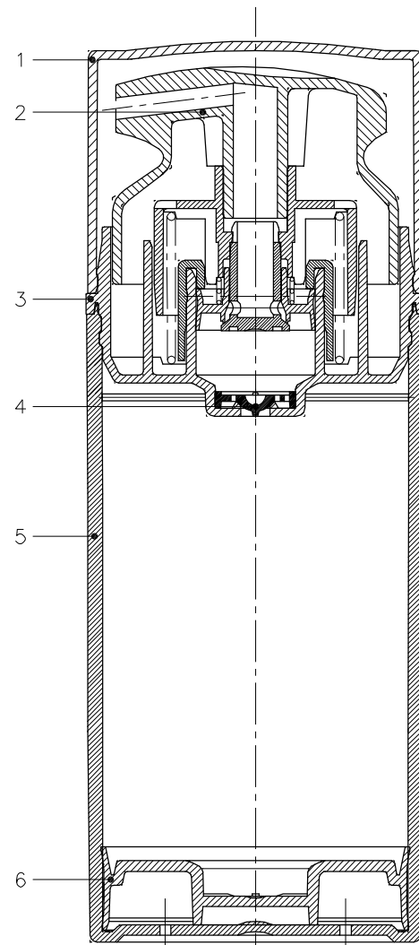
SECTION A-A'
