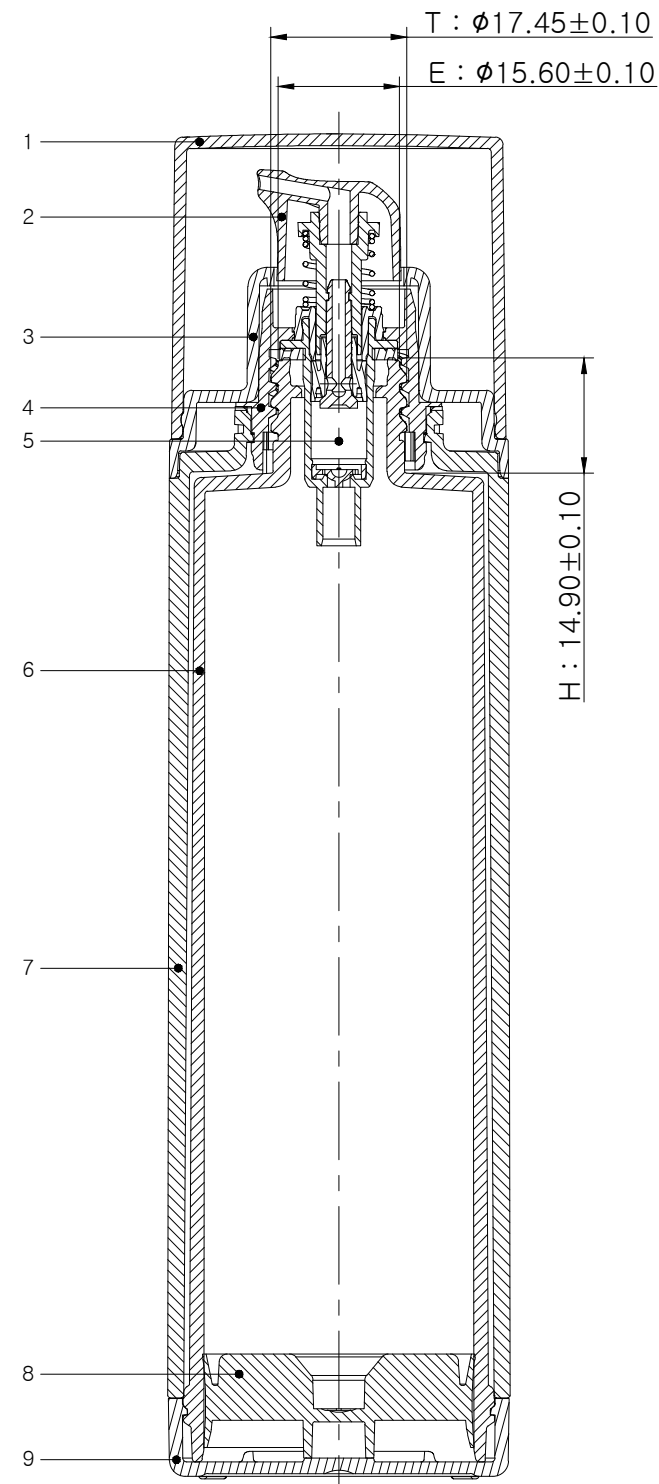
SECTION A-A'
