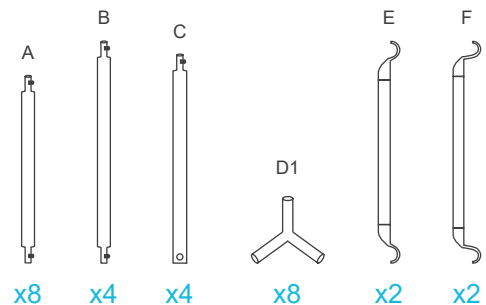
TEILE STAHLRAHMEN
