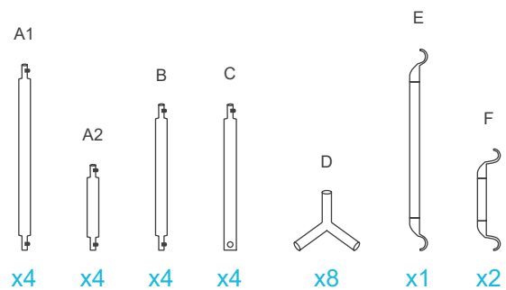
TEILE STAHLRAHMEN
