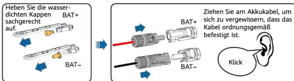
Akkuklemmen (BAT+/BAT-)
