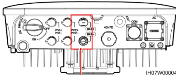
Akkuklemmen (BAT+/BAT-)
