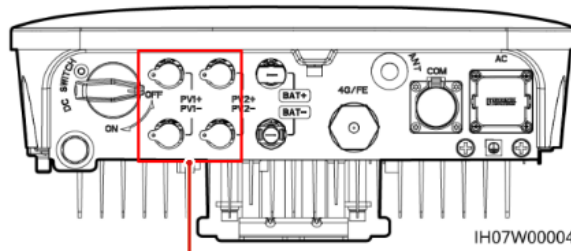
DC-Eingangsklemmen
