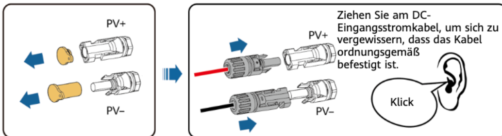
DC-Eingangsklemmen
