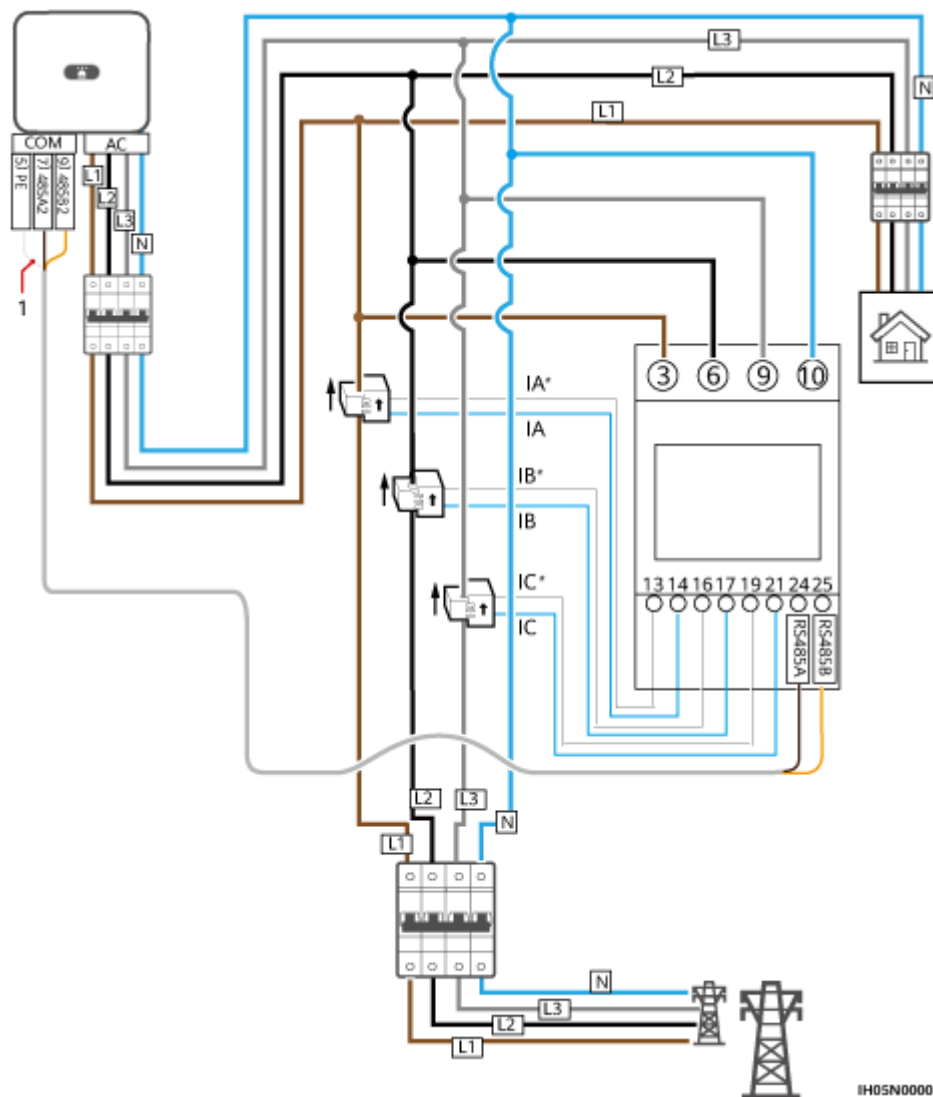
Abbildung 5-24 Dreiphasige vieradrige Verbindung (Smart Dongle-Vernetzung)
