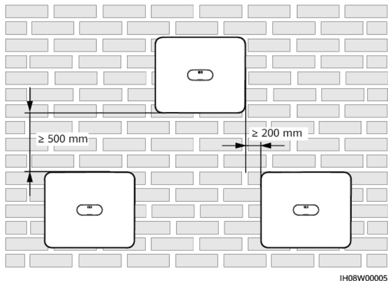
Abbildung 4-4 Dreiecks-Installationsmodus (empfohlen)
