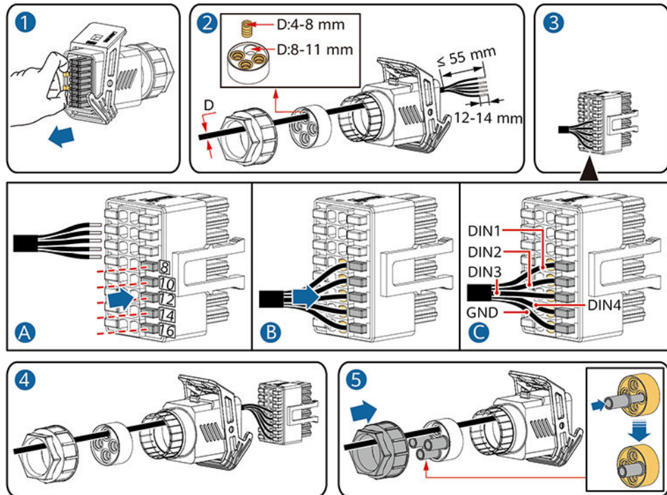
Abbildung 5-40 Kabelmontage
