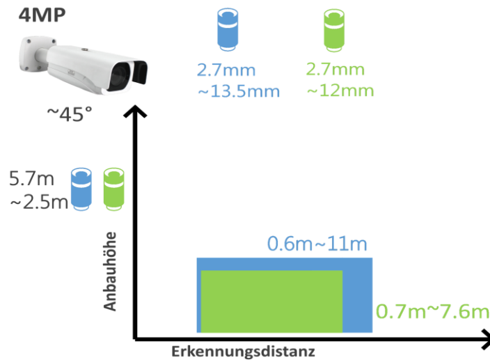
Abbildung 3: Detektionsreichweiten, können durch Umgebungseinflüsse variieren
