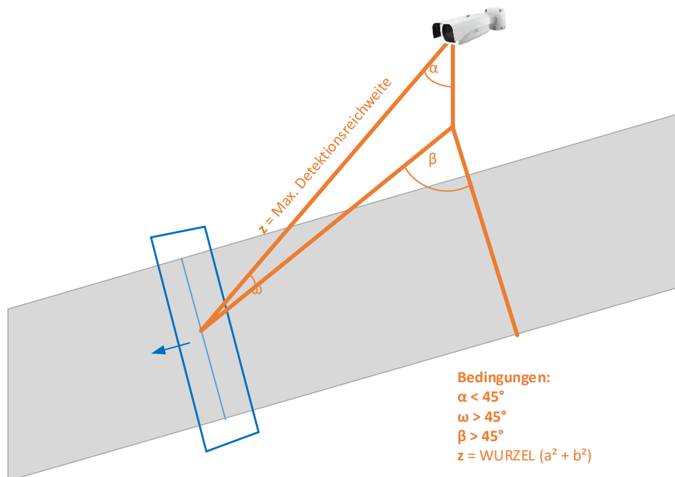
Abbildung 2: Detektionswinkel und max. Entfernung
