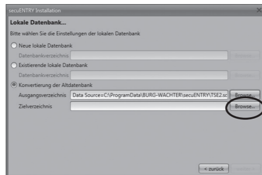
Abb. 35: Verzeichnis- und Passworteingabe
