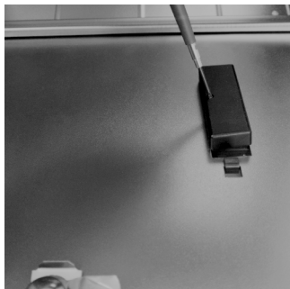
Abbildung 3: Batteriefachdeckel öffnen
