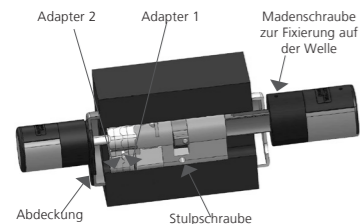
Schematische Darstellung des Zylinders
