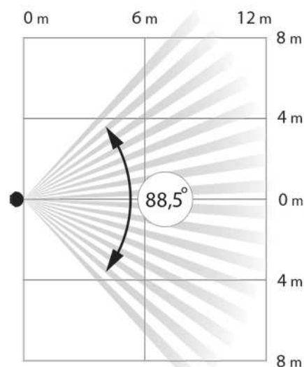
Angles de vue horizontaux et verticaux du détecteur
