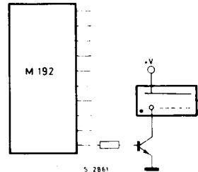
Fig. 5 - Gas discharge readout
