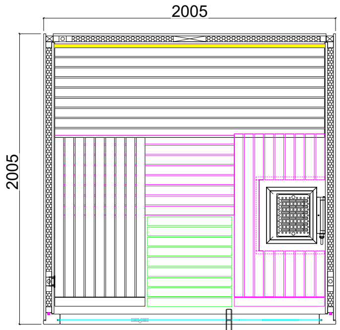
Aufbau rechts
