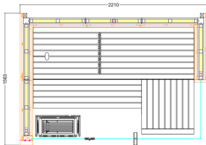
Aufbau links
