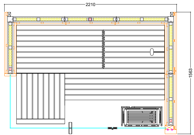
Aufbau rechts
