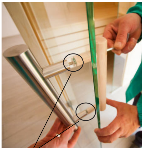
Inserir a anilha plana de plástico no puxador de aço inoxidável
