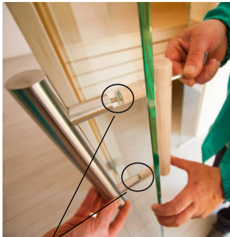
Włóż podkładkę z tworzywa sztucznego do uchwytu Niroy
