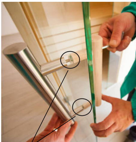
Pose des rondelles de calage en plastique pour poignée inox
