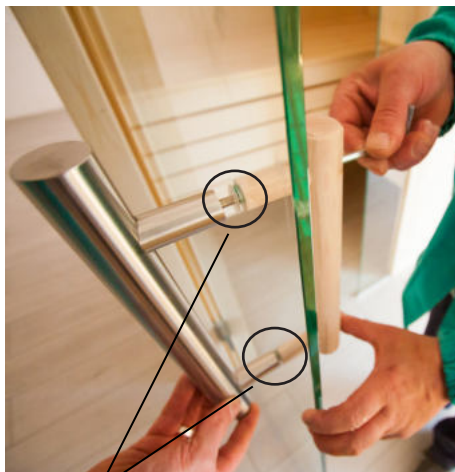
Kunststoff Beilagscheibe bei Niro-Griff beilegen
