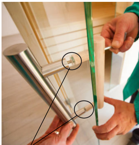
Applicare rondelle di plastica nelle maniglie Nirosta
