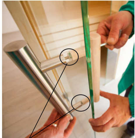
Kunststoff Beilagscheibe bei Niro-Griff beilegen
