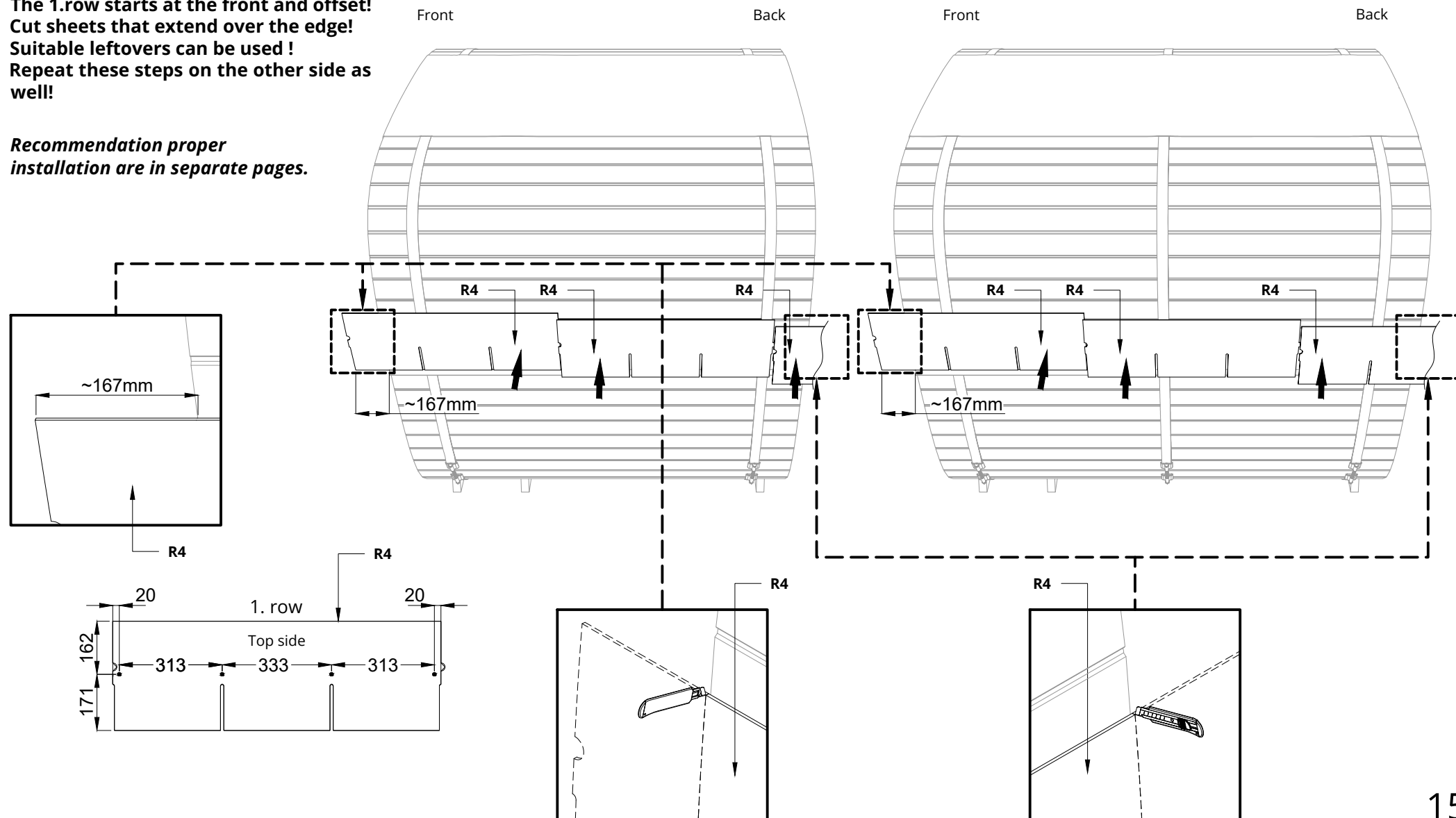
Dice Sauna (COMFY2.0)
