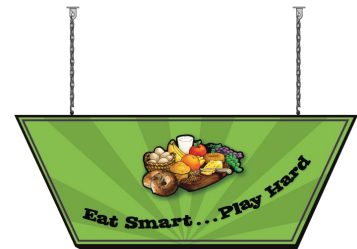
Right Message
