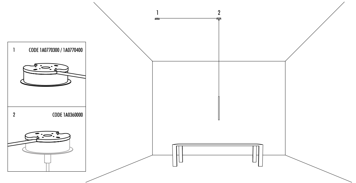
1A0770300 / 1A0770400 - KIT ROSONE + DECENTRATORE / KIT CEILING ROSE + DECENTRALIZER | 1A0360000 KIT DECENTRATORE / DECENTRALIZATION KIT
