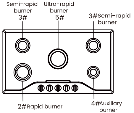
PRO GH2905SS2FC
