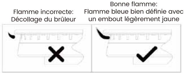
Fig.22 (Modèles de bonne et de mauvaise flammes)
