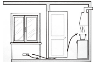
Élargissement un orifice de ventilation entre la fenêtre et le plancher.
