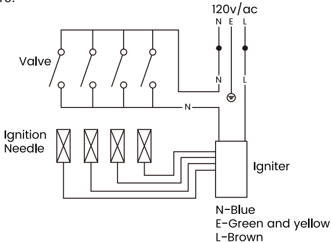
PRO GH2304SS/ES Fig.19
