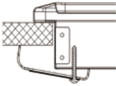
Position de l'accroche pour H=0.8" supérieur
