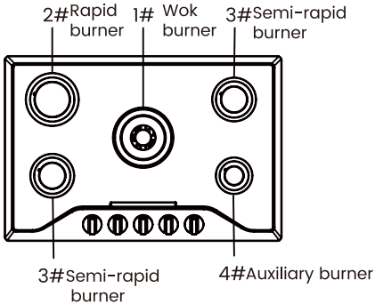
PRO GH2305SF/EF PRO GH3305SF/EF
