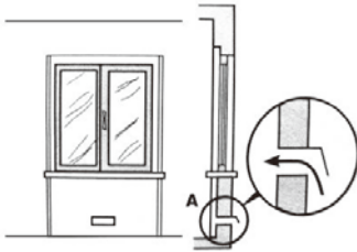
Exemples des trous de ventilation pour l'air comburant.
