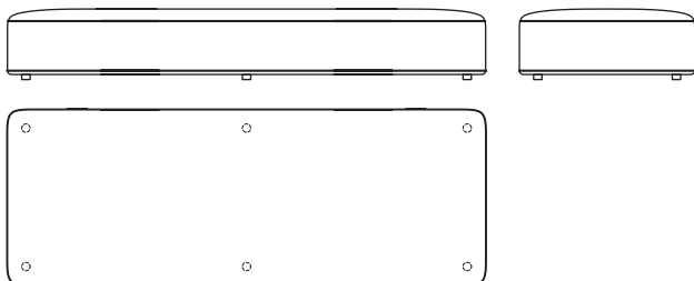
12002-43 Causeway module 3 W2850 D1050 H420
