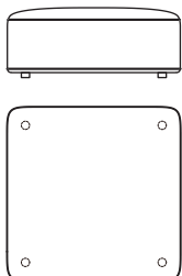
12002-41 Causeway module 1 W1050 D1050 H420
