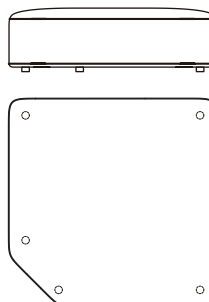
12002-45 Causeway module 5 W1380 D1050/1380 H420
